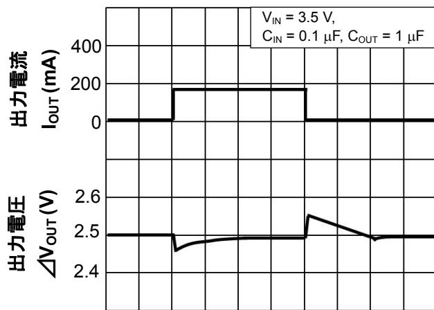
V_{OUT}=2.5V (I_{OUT} = 1mA \Leftrightarrow 150mA)
