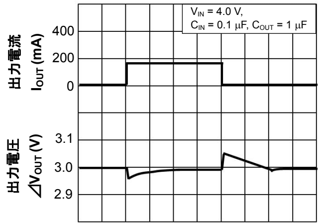
V_{OUT}=3.0V (I_{OUT} = 1mA \Leftrightarrow 150mA)
