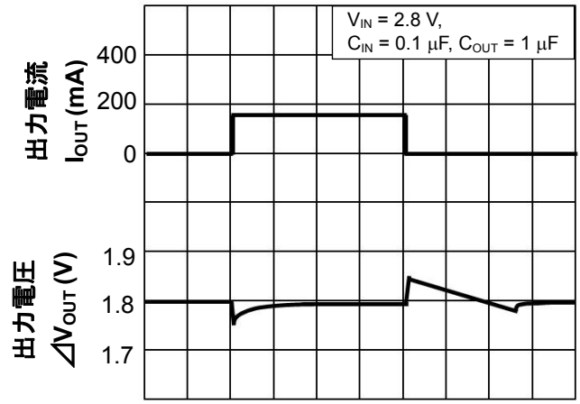
V_{OUT}=1.8V (I_{OUT} = 1mA \Leftrightarrow 150mA)
