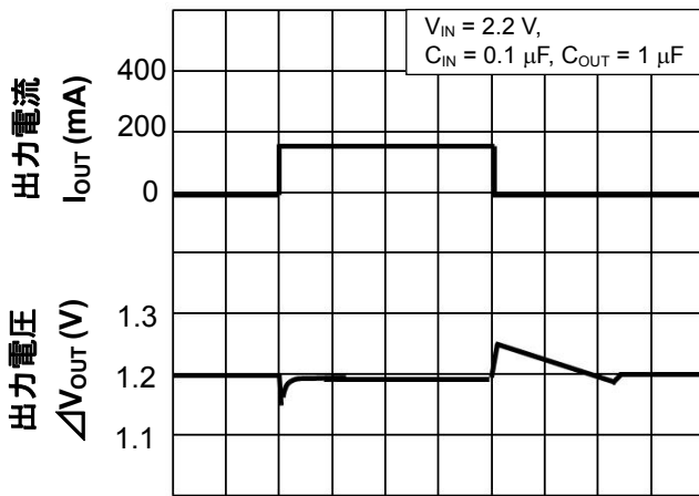
V_{OUT}=1.2V (I_{OUT} = 1mA \Leftrightarrow 150mA)
