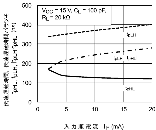
図 12.2.11 t_{pHL}, t_{pLH}, |t_{pLH} - t_{pHL}| - I_F
