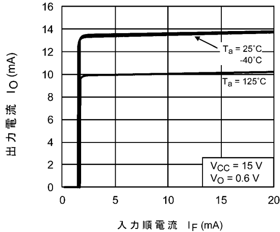
図 12.2.7 I_O - I_F
