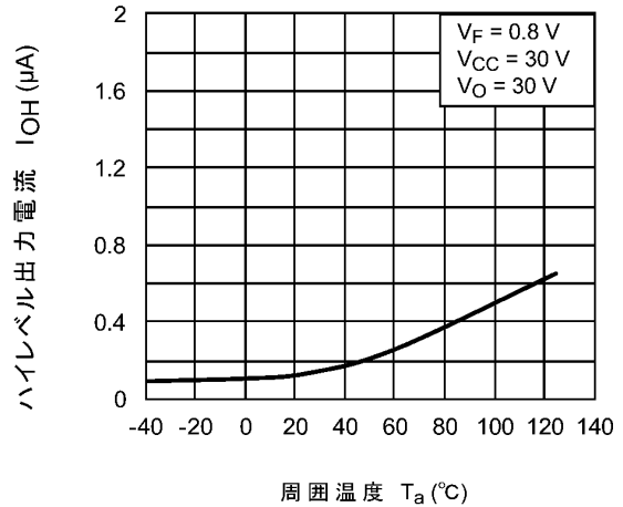
図 12.2.8 I_{OH} - T_a
