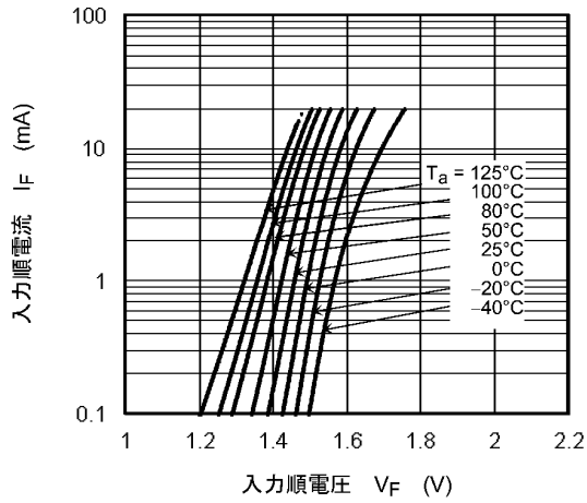
図 12.2.1 I_F - V_F
