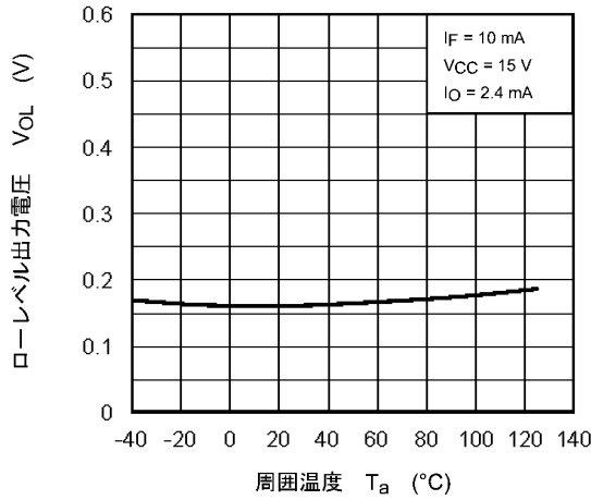
図 12.2.9 V_{OL} - T_a
