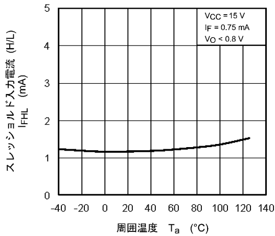
図 12.2.3 I_{FHL} - T_a
