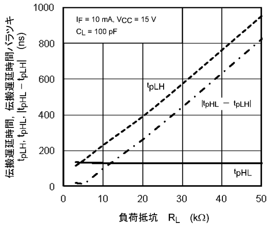
図 12.2.13 t_{pLH}, t_{pHL}, |t_{pHL} - t_{pLH}| - R_L
