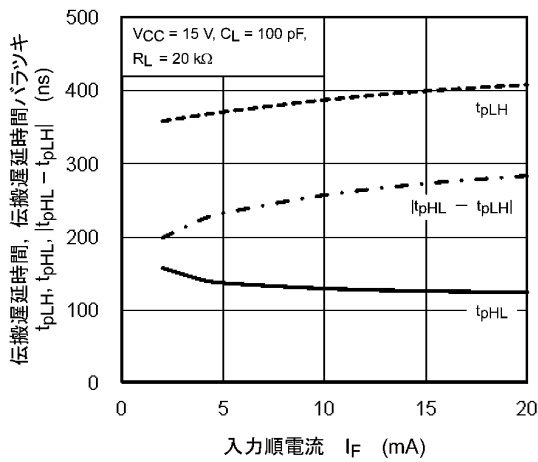
図 12.2.11 t_{pLH}, t_{pHL}, |t_{pHL} - t_{pLH}| - I_F
