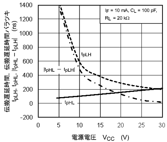
図 12.2.12 t_{pLH}, t_{pHL}, |t_{pHL} - t_{pLH}| - V_{CC}
