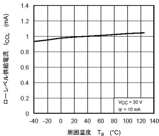
図 12.2.5 I_{CCL} - T_a
