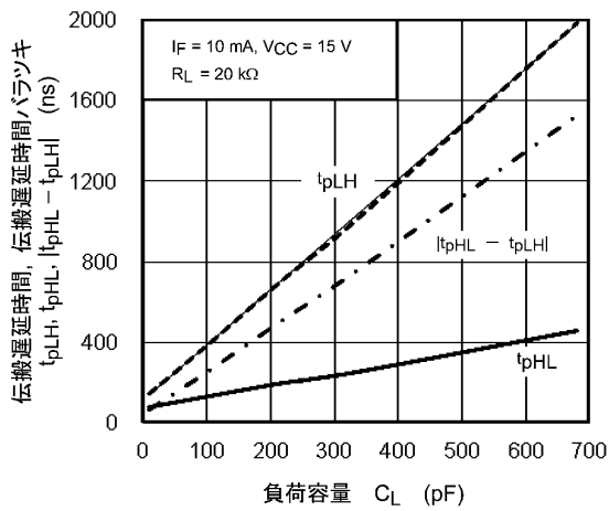
図 12.2.15 t_{pLH}, t_{pHL}, |t_{pHL} - t_{pLH}| - C_L
