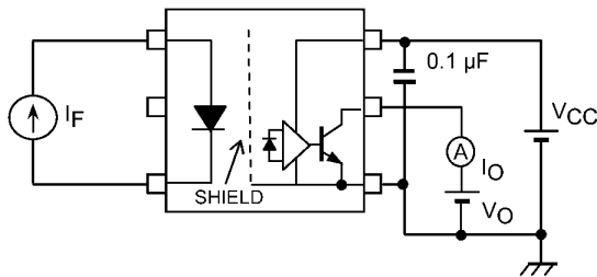
図 12.1.5 I O 測定回路
