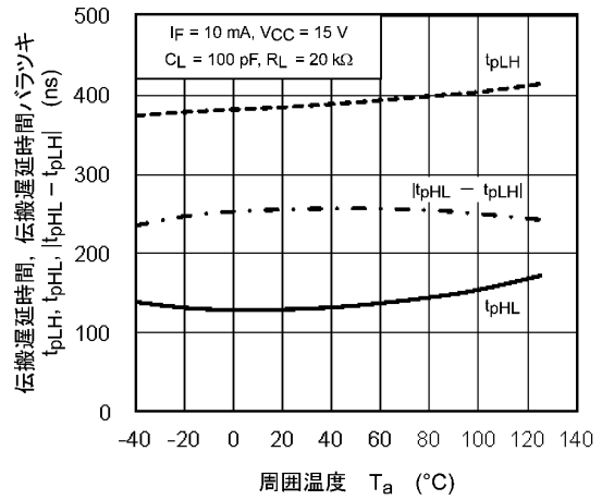
図 12.2.10 t_{pLH}, t_{pHL}, |t_{pHL} - t_{pLH}| - T_a
