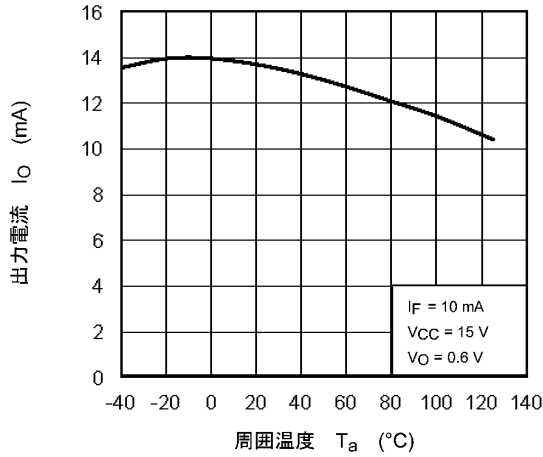
図 12.2.7 I_O - T_a
