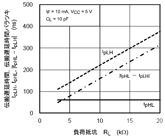
図 12.2.14 t_{pLH}, t_{pHL}, |t_{pHL} - t_{pLH}| - R_L
