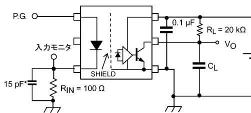
図 12.1.6 伝搬遅延時間測定回路, 波形
