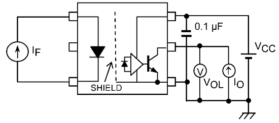
図 12.1.2 V OL 測定回路
