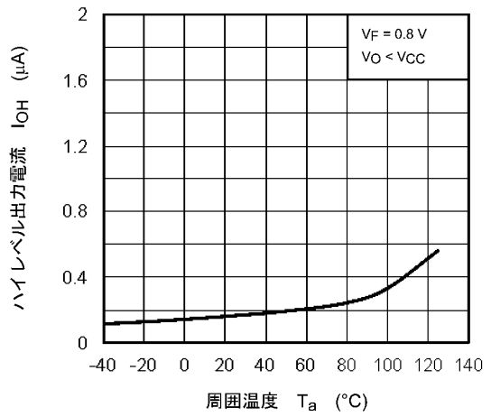
図 12.2.4 I_{OH} - T_a
