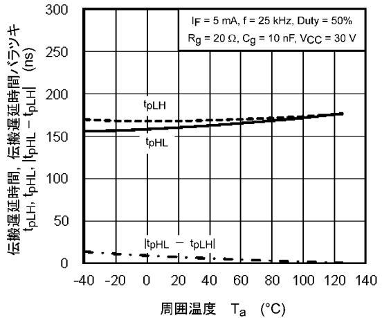
図 13.2.12 t_{pLH}, t_{pHL}, |t_{pHL} - t_{pLH}| - T_a
