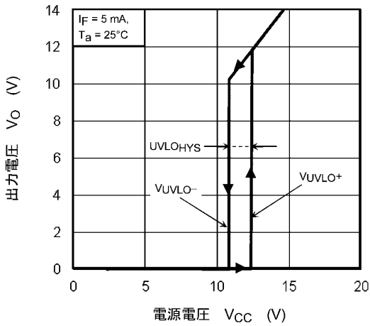
図 13.2.11 V_o(V_{UVLO}) - V_{CC}
