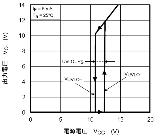
図 12.2.11 V_o(V_{UVLO}) - V_{CC}
