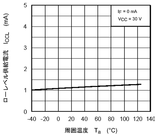
図 12.2.5 I_{CCL} - T_a
