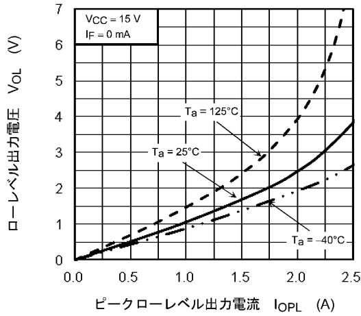
図 12.2.9 V_{OL} - I_{OPL}
