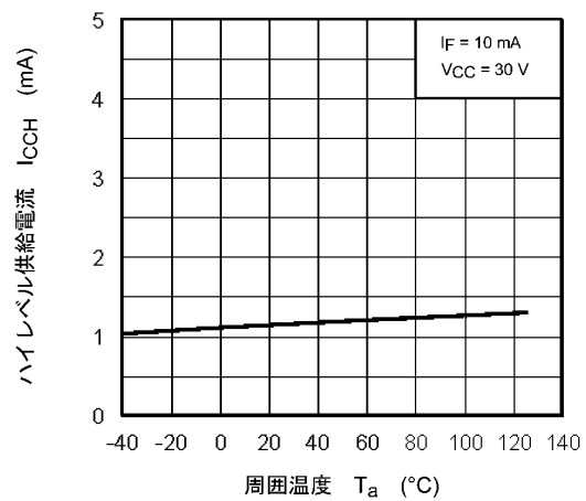
図 12.2.6 I_{CCH} - T_a
