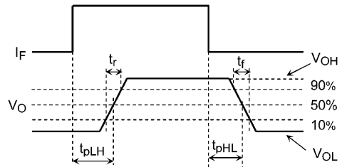
図 12.1.7 伝搬遅延時間測定回路, 波形
