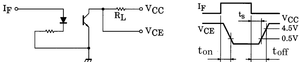
図 1: スwitchング時間測定回路
