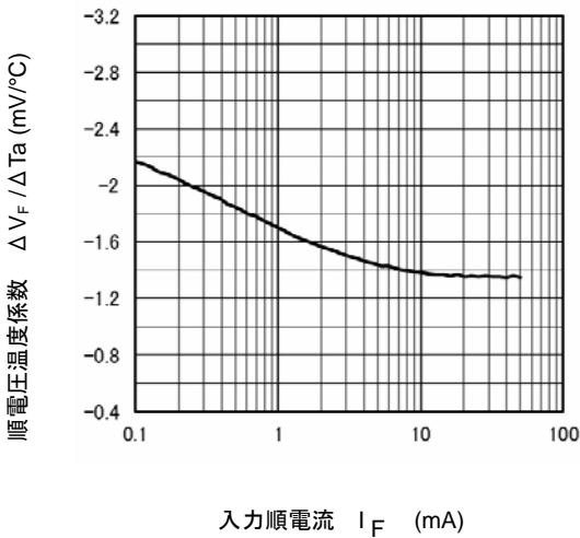
\Delta V_F / \Delta T_a - I_F
