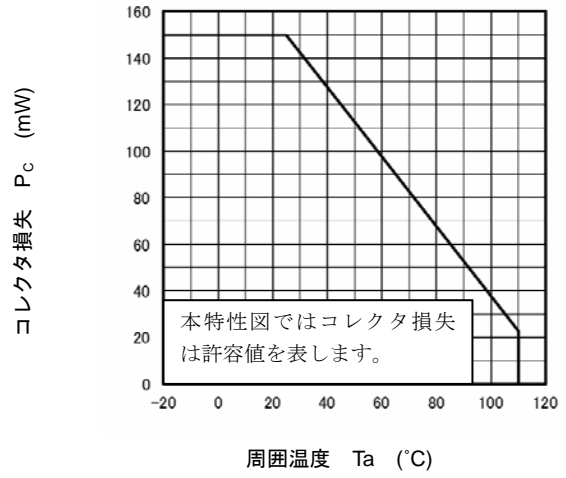
P_C - T_a
