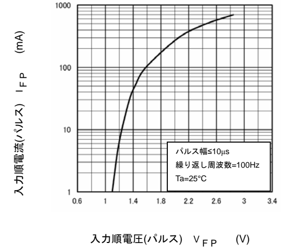
I_{FP} - V_{FP}
