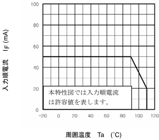
I_F - T_a
