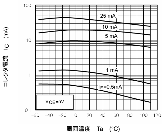
I_C - T_a
