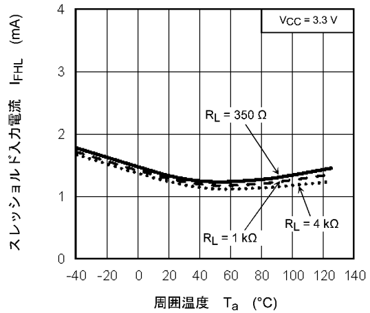
図 13.2.8 I_{FHL} - T_a
