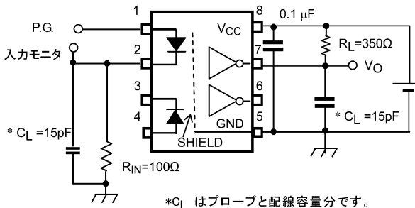
図 13.1.5 伝搬遅延時間測定回路, 波形
