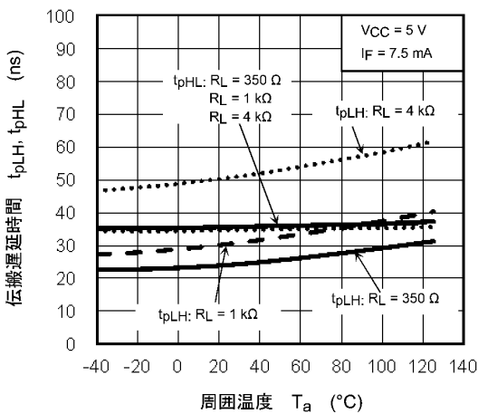
図 13.2.11 t_{pLH} / t_{pHL} - T_a
