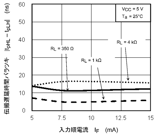
図 13.2.16 |t_{pHL} - t_{pLH}| - I_F
