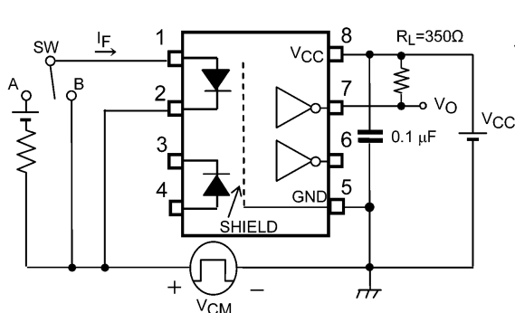
図 13.1.6 コモンモードノイズ除去電圧測定回路, 波形
