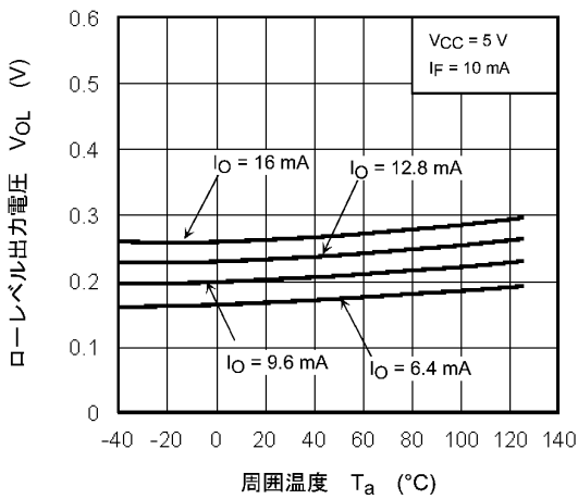
図 13.2.3 V_{OL} - T_a
