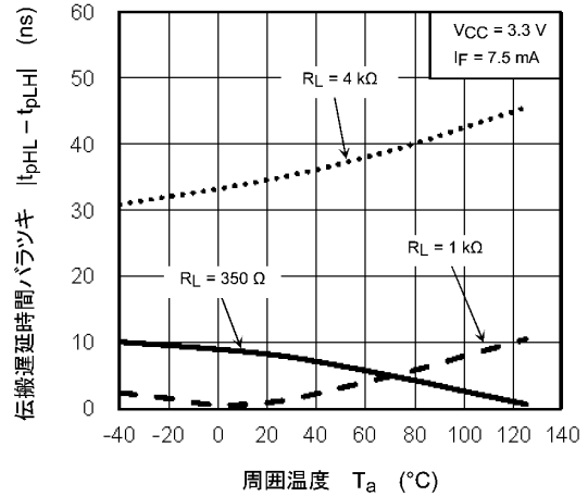
図 13.2.14 |t_{pHL} - t_{pLH}| - T_a
