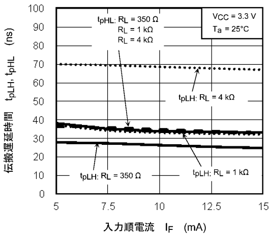
図 13.2.17 t_{pLH} / t_{pHL} - I_F
