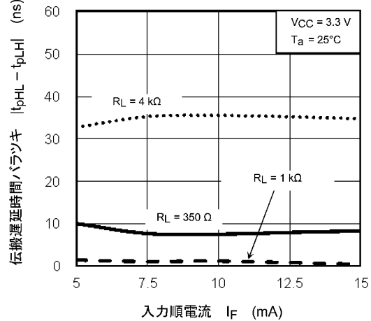
図 13.2.18 |t_{pHL} - t_{pLH}| - I_F
