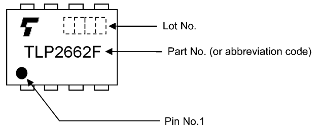
図 16.2 TLP2662F
