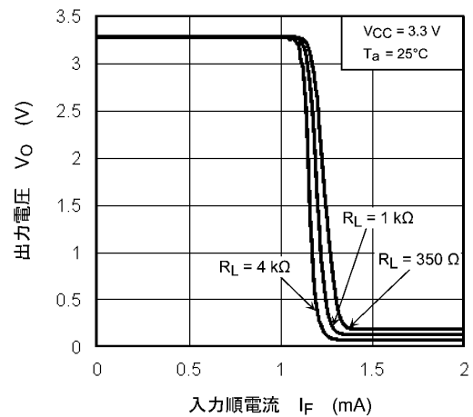
図 13.2.6 V_O - I_F
