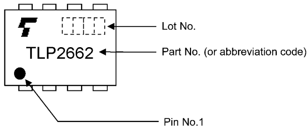
図 16.1 TLP2662
