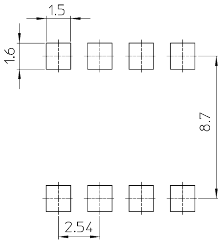
図 15.1 (LF1), (LF5)タイプ (unit:mm)
