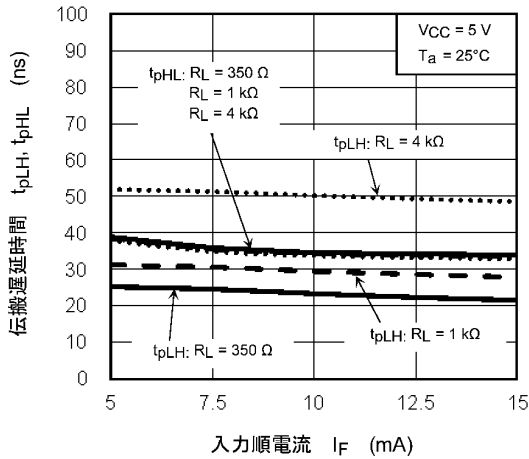
図 13.2.15 t_{pLH} / t_{pHL} - I_F
