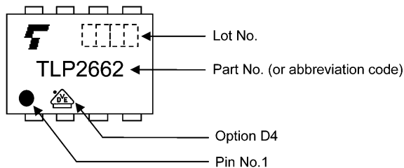
図 17.3 TLP2662 表示例
