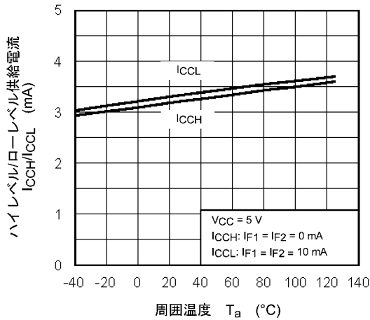
図 13.2.9 I_{CCH} / I_{CCL} - T_a
