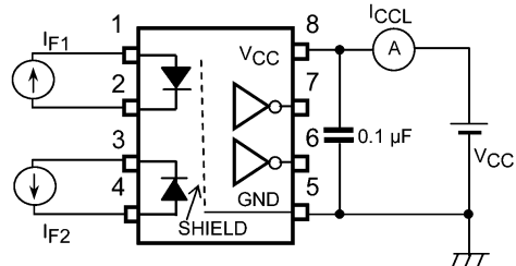
図 13.1.4 I CCL 測定回路
