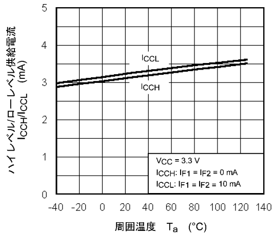
図 13.2.10 I_{CCH} / I_{CCL} - T_a
