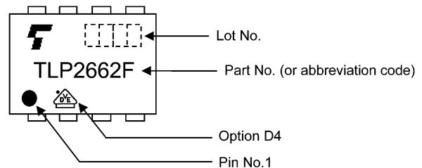
図 17.4 TLP2662F 表示例
