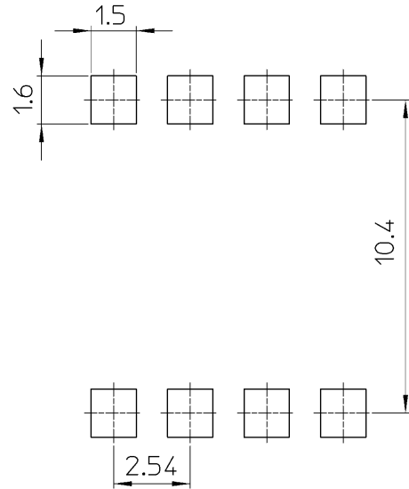
図 15.2 (LF4)タイプ (unit:mm)
