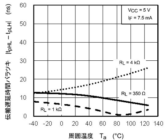
図 13.2.12 |t_{pHL} - t_{pLH}| - T_a
