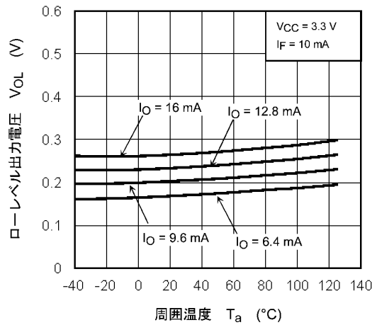
図 13.2.4 V_{OL} - T_a
