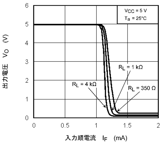
図 13.2.5 V_O - I_F
