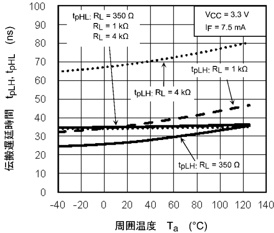
図 13.2.13 t_{pLH} / t_{pHL} - T_a
