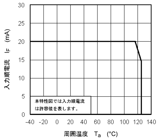
図 13.2.2 I_F - T_a
