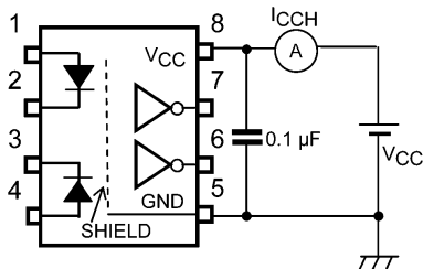
図 13.1.3 I CCH 測定回路
