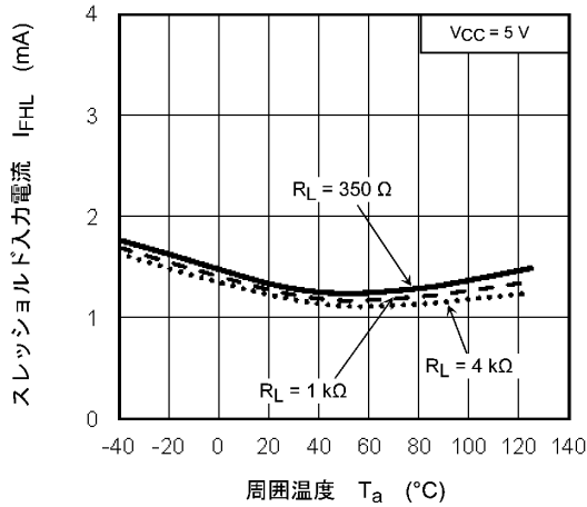
図 13.2.7 I_{FHL} - T_a
