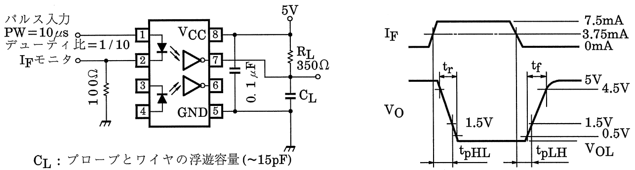
図 1. t_{pHL} 、 t_{pLH} 測定回路、波形
