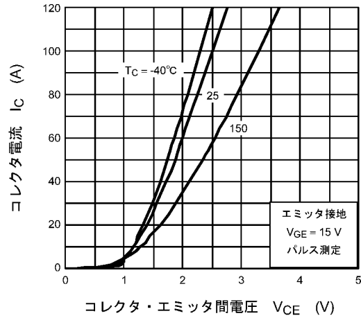
図 8.4 I_C - V_{CE}
