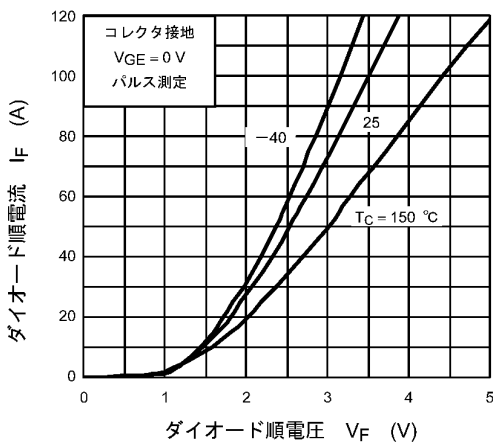
図 8.11 I_F - V_F
