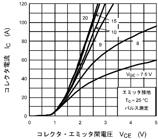
図 8.2 I_C - V_{CE}
