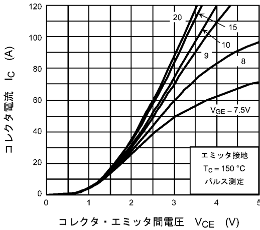
図 8.3 I_C - V_{CE}
