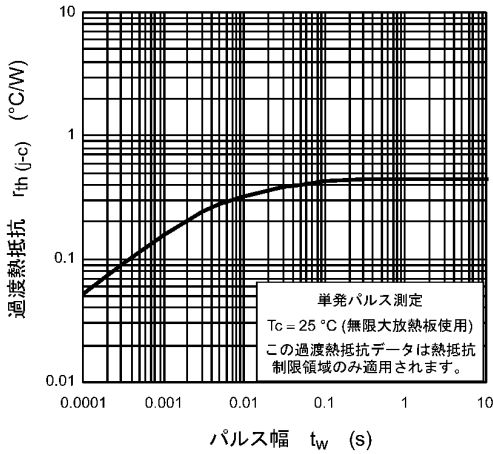
図 8.9 r_{th(j-c)} - t_w (最大値 (保証値))
