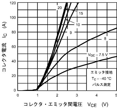
図 8.1 I_C - V_{CE}
