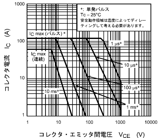
図 8.10 安全動作領域 (最大値 (保証値))
