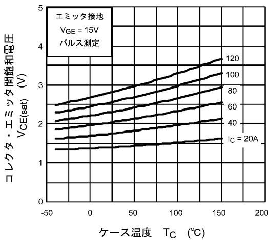
図 8.5 V_{CE(sat)} - T_C
