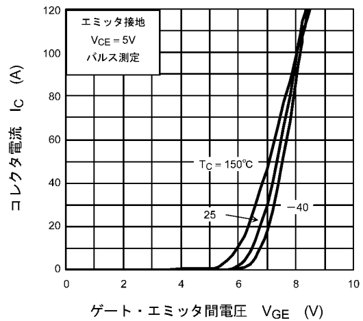
図 8.6 I_C - V_{GE}
