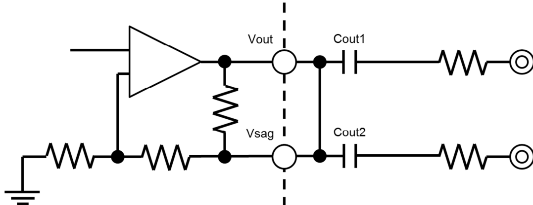
(B)出力コンデンサを2つにする場合
