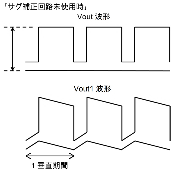
Vout 端子と Vout1 端子の波形
