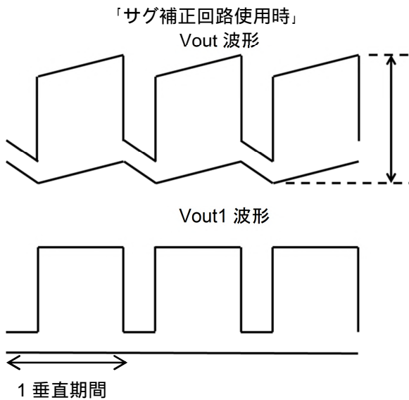
Vout 端子と Vout1 端子の波形
